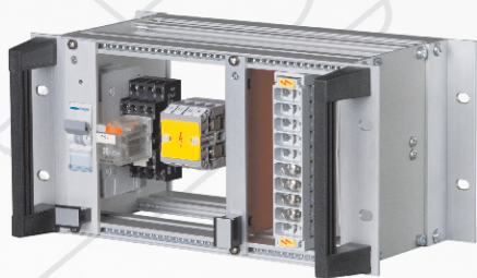
Kaseta DIN 35
